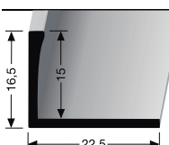
306 U ∅ 15 mm ungestanzt
