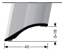
247 SK selbstklebend
