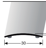
451 SK selbstklebend
