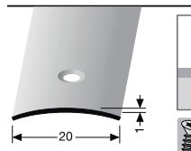
471 mittig versenkt gebohrt
