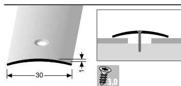
451 mittig versenkt gebohrt
