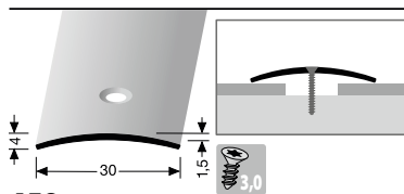
459 mittig versenkt gebohrt
