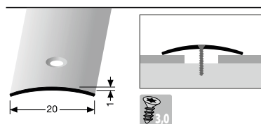
471 mittig versenkt gebohrt
